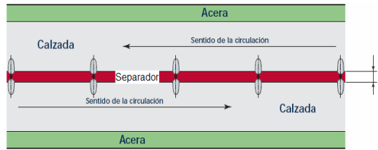
Figura 510.65c) Disposición Central doble (para 1,5\text{ m} \geq b \leq 4\text{ m} )
