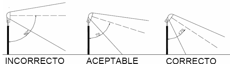
Figura 570.7.e) ángulos de inclinación de proyectores
